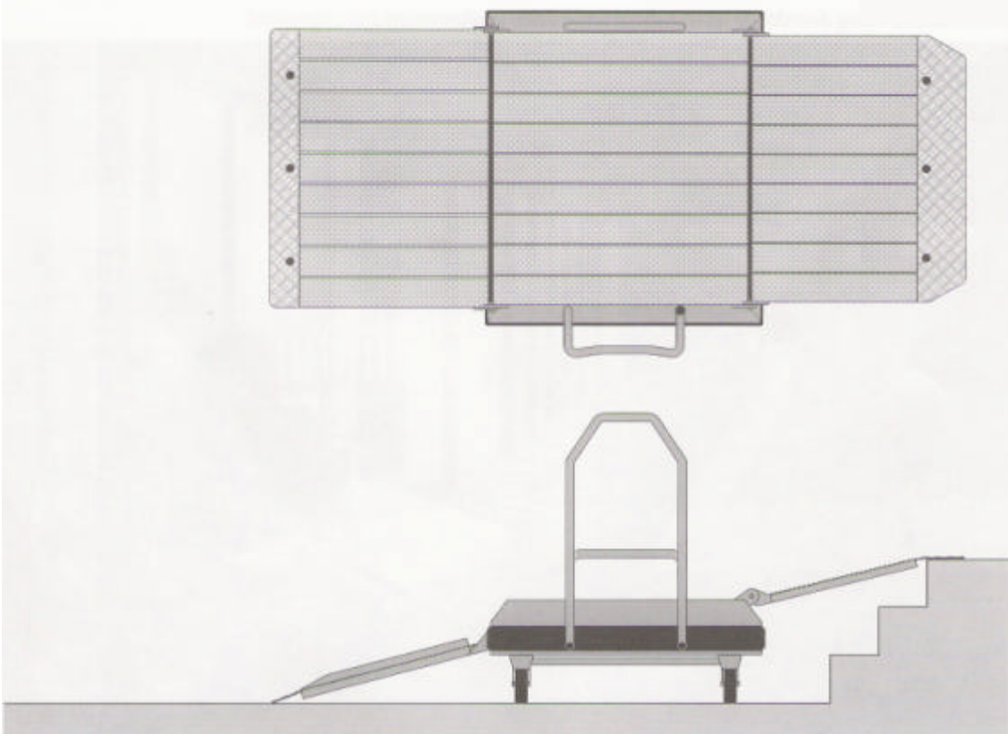
Vlinderklapbrug (bovenaanzicht).
